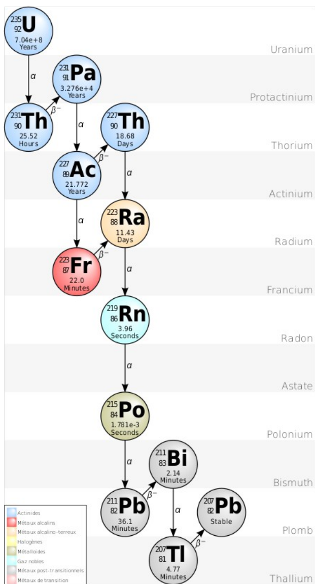
Famille radioactive de l'actinium.
